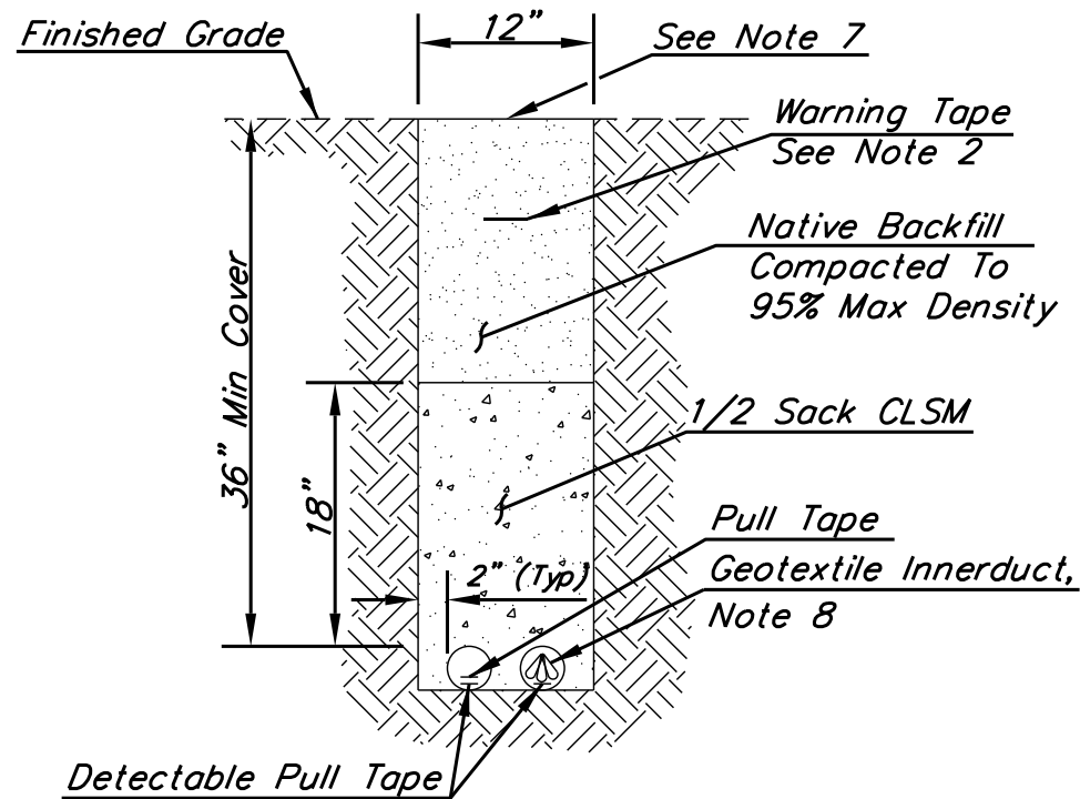
2-3" CONDUIT TRENCH DETAIL
